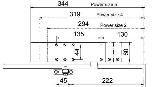
Fig2 - Opp hinge right
